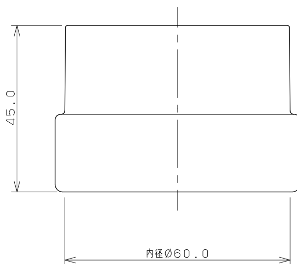
50Aソケット
