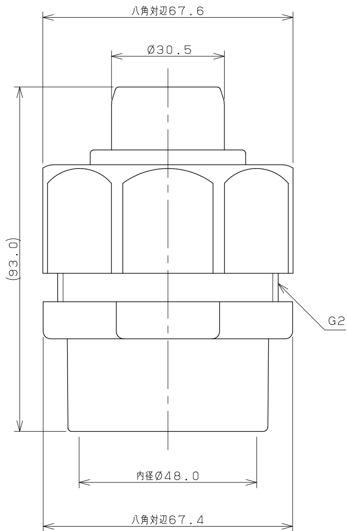
50Aソケット
