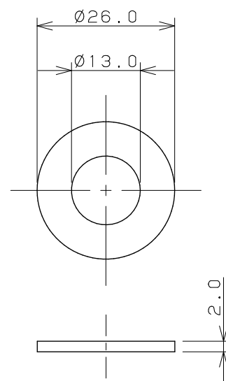
パッキン×4
