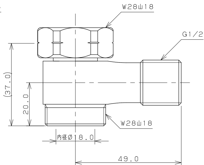
分岐継手
