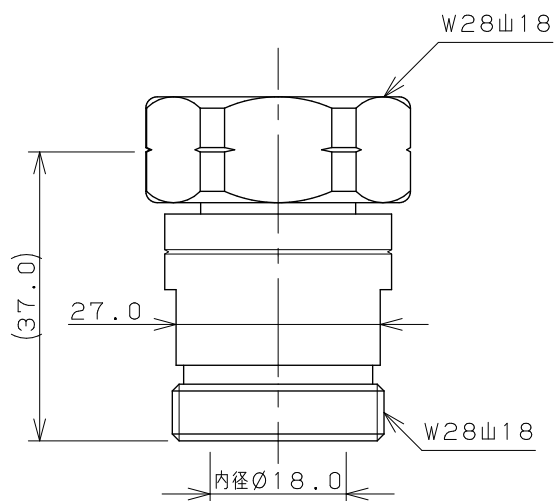
延長継手
