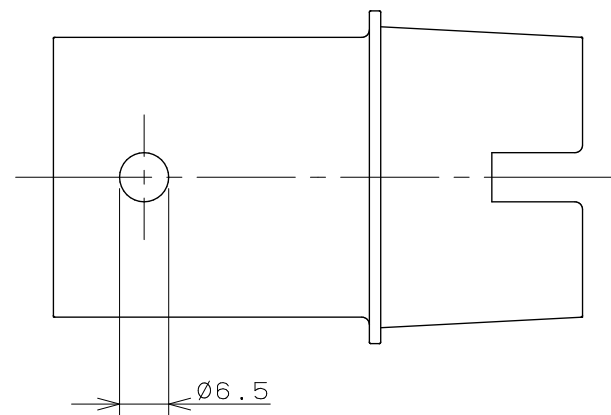
締付工具
