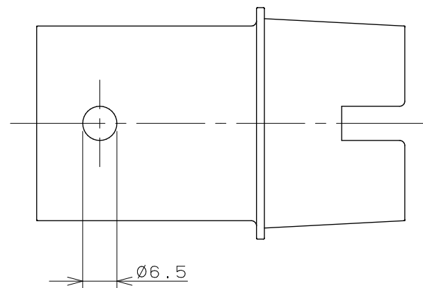
締付工具
