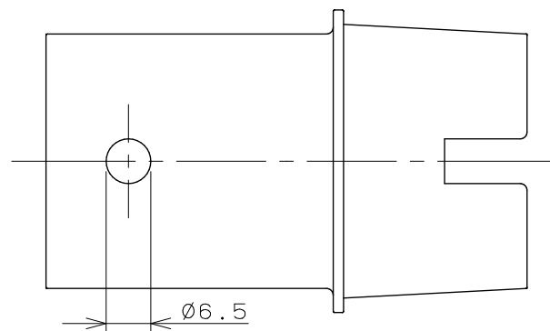
締付工具
