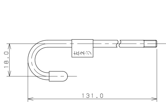
フック棒
