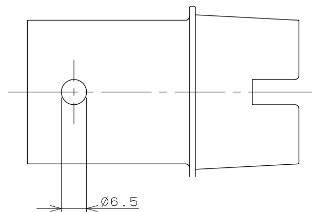
締付工具
