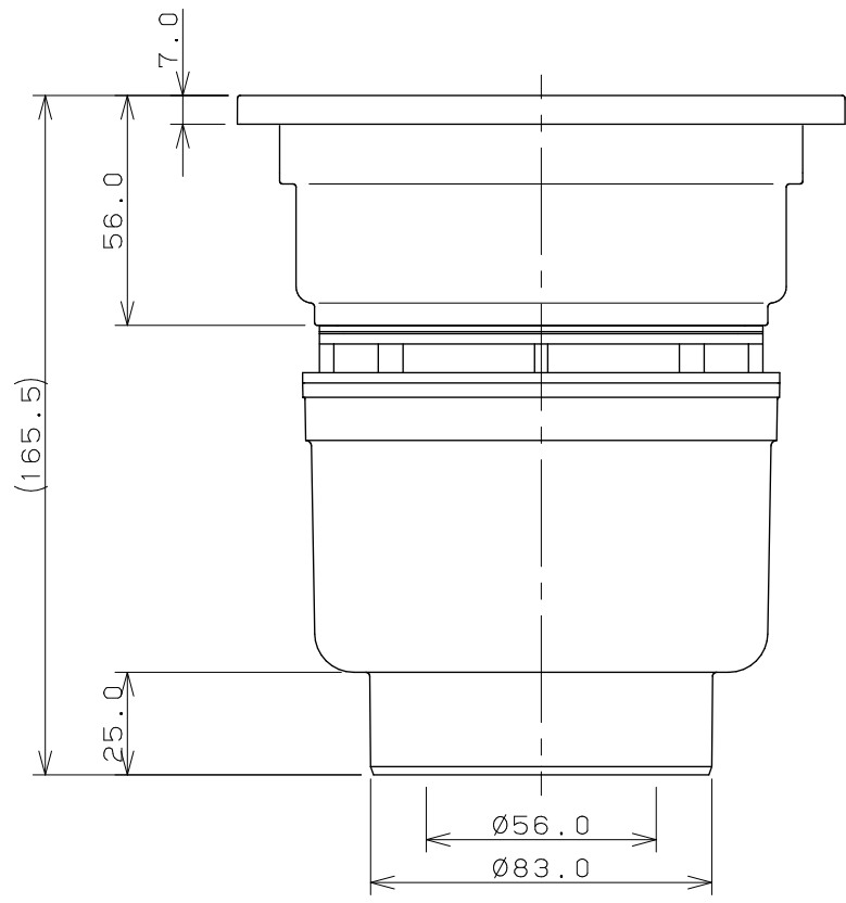
締付金具 (尺度 1/3)
