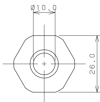
ナット
