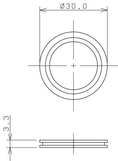
リング
