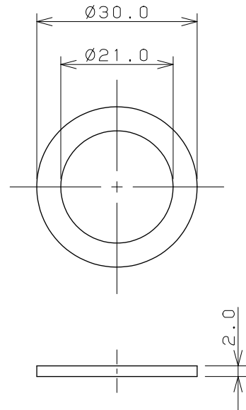
パッキン
