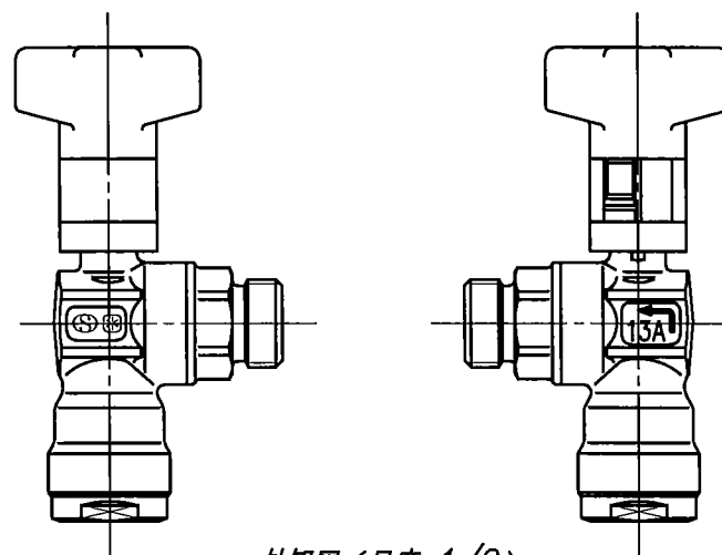
外觀図 (尺度 1/2)
