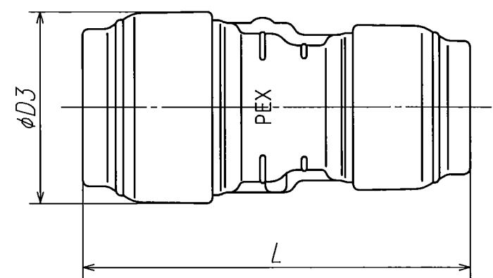
外觀図
