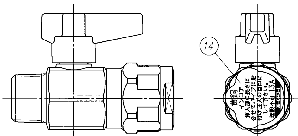
外観図
