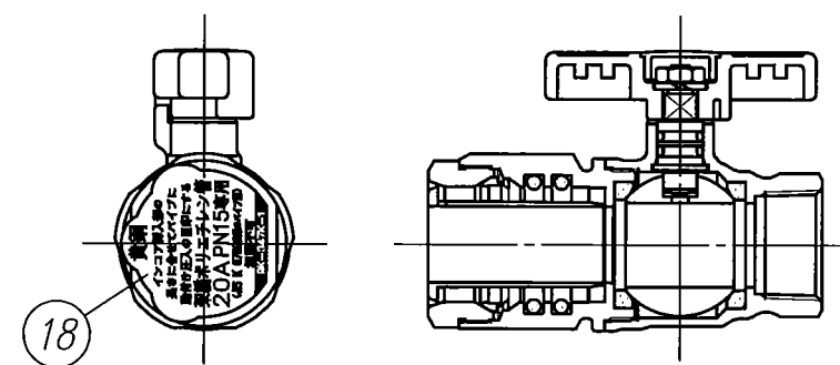
包装時組付図 (尺度 1/2)
