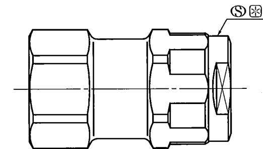
外観図
