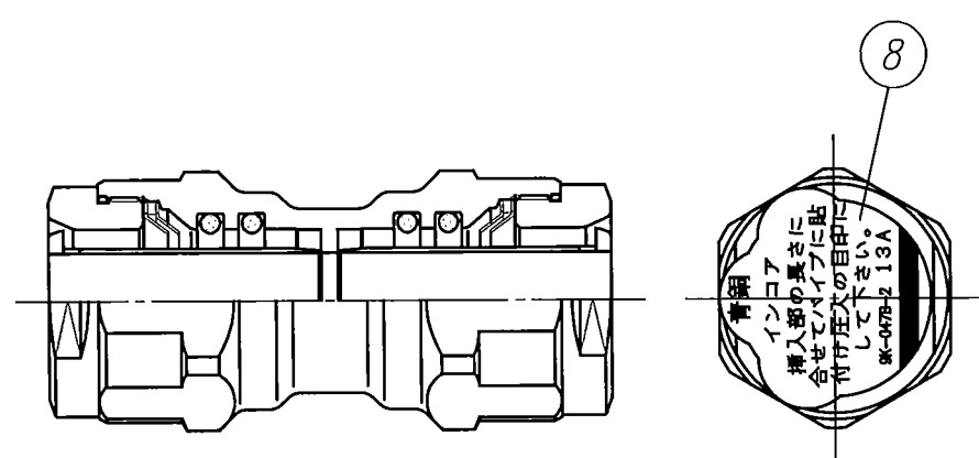
包装時組付図
