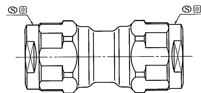
外觀図
