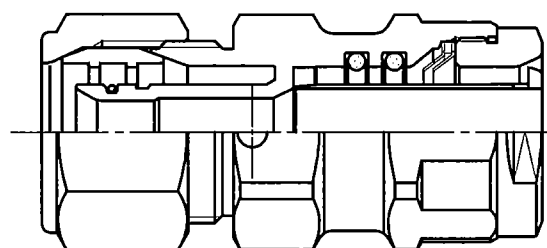
包装時組付図
