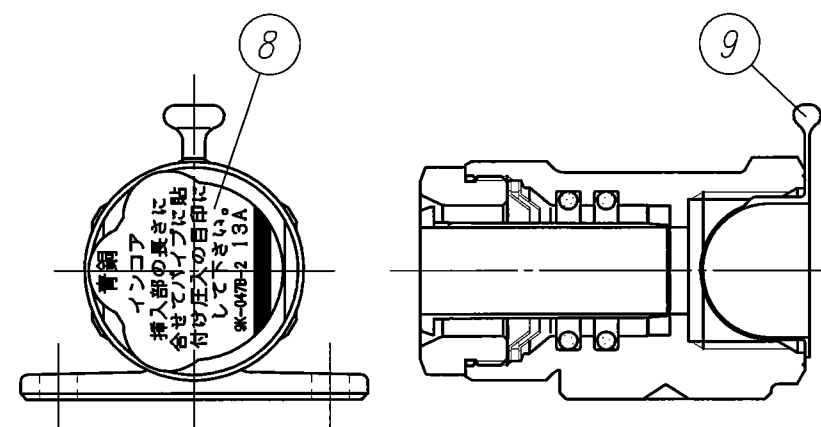
包装時組付図
