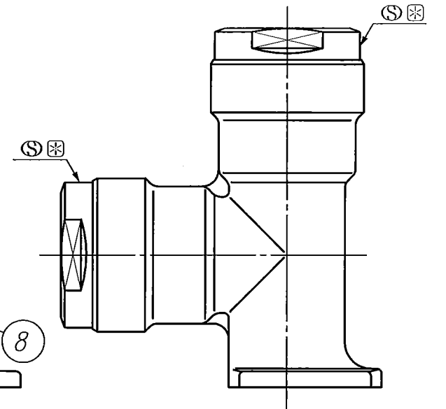
外觀図
