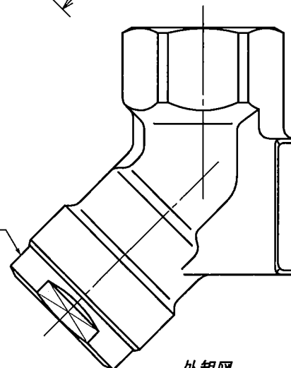
外觀図
