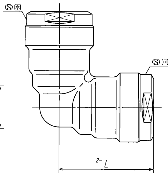
外観図
