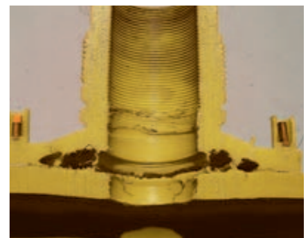
冷却時間を守らずに穿孔
