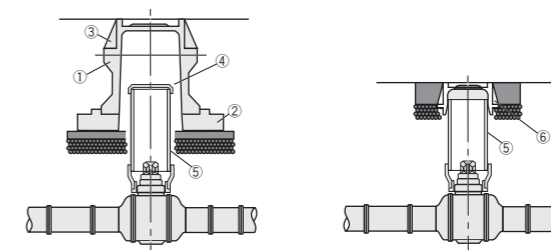
車両重量を受ける場所(本支管等) 車両重量を受けない場所(内管等)
