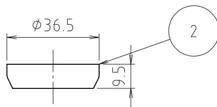
寸法 30
