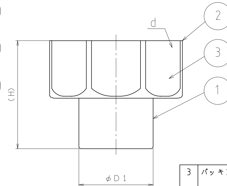
寸法 38×2
