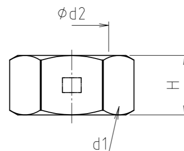
寸法 20
